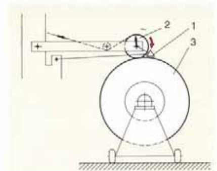
Bild 35: Dockenwickler zu Kalandrierung in einem Textilveredlungs-Betrieb.
