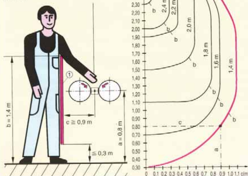
Bild 24: Schutzzaun (1) für den Normalbetrieb. Damit verhindert wird, dass die Gefahrenstellen mit den oberen Gliedmassen erreicht werden können, müssen die Sicherheitsabstände gemäss EN 294, Tabelle 2, eingehalten werden.
