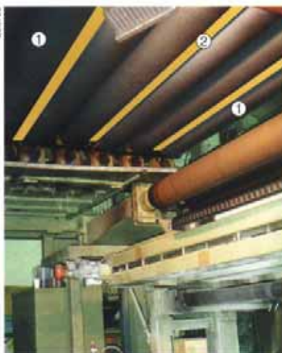
Bild 20: Kalender in einem Kunststoffverarbeitenden Betrieb. Die Einlaufstellen an den Kühlwalzen (1) sind mit der Hand erreichbar und deshalb mit Schutzstangen (2) gesichert.
