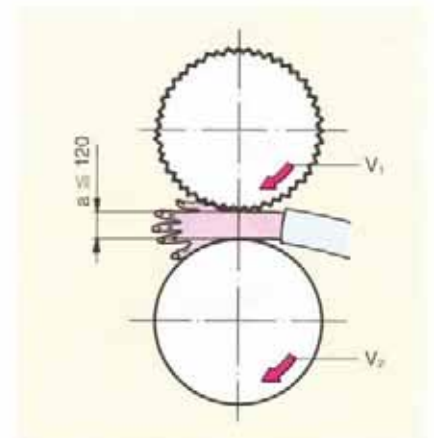
Bild 7: Walzenpaar mit einem Spalt von höchstens 120 mm zwischen den Walzen. Die Oberfläche der einen Walze weist eine grosse Reibungskraft auf. Es besteht Einzugsgefahr für Finger, Hände und Arme.
