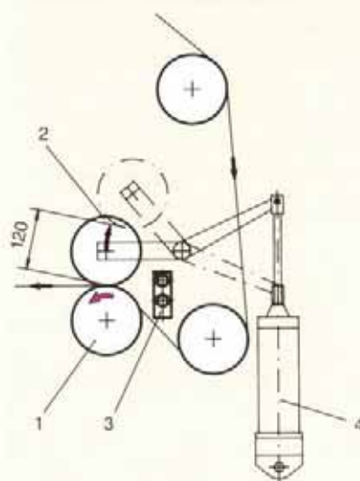
Bild 35: Dockenwickler zu Kalandrierung in einem Textilveredlungs-Betrieb.
