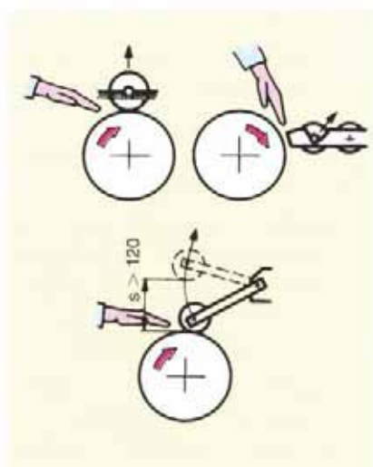
Bild 12: Vermeiden der Einzugsgefahr für Finger und Hände durch:
