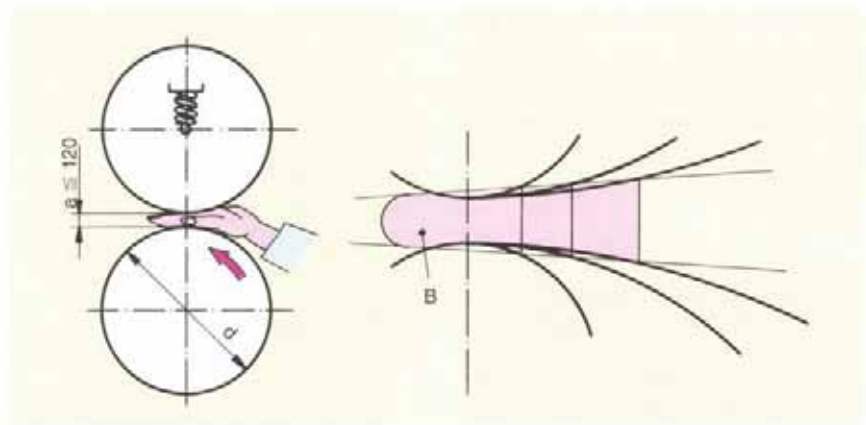
Bild 3: Walzenpaar mit beschränkt nachgiebigem Lager.
