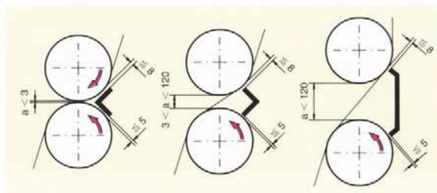
Bild 16: Schutzstangen und Schutzprofile zum Sichern von Einzugsstellen.
