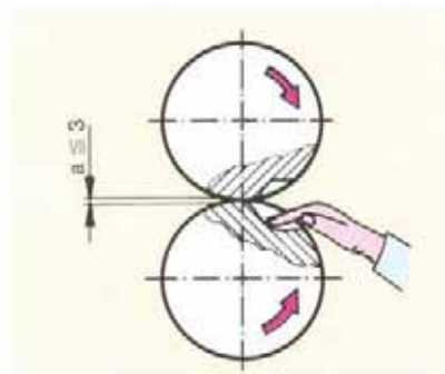
Bild 2: Walzenpaar mit Vertiefung in der Oberfläche.
