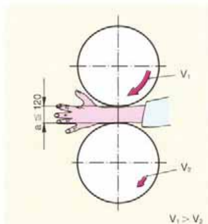
Bild 6: Walzenpaar mit einem Spalt von höchstens 120 mm zwischen den Walzen. Die Umfangsgeschwindigkeit der einen Walze ( V_1 ) ist grösser als diejenige der anderen Walze ( V_2 ). Es besteht Einzugsgefahr für Finger, Hände und Arme.
