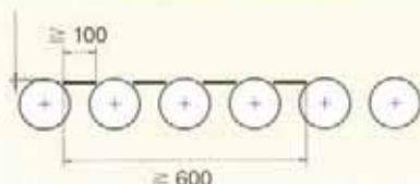
Bild 40: Übergang über eine Rollenbahn in einer Spedition.
