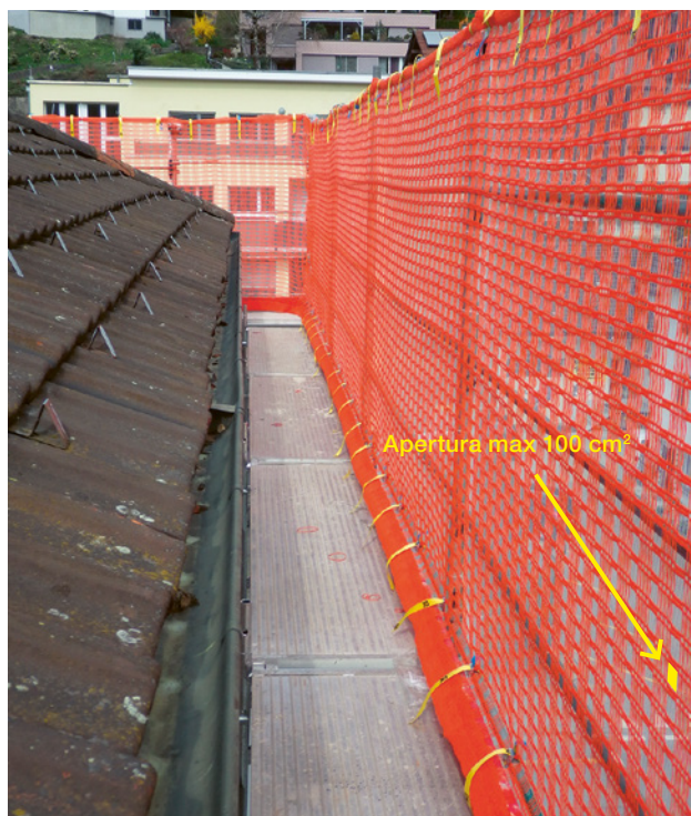
1 Parete di protezione da copritetto corretta e testata secondo la norma SN EN 13374 con rete che delimita il ponte da lattoniere e cinghie di fissaggio.
