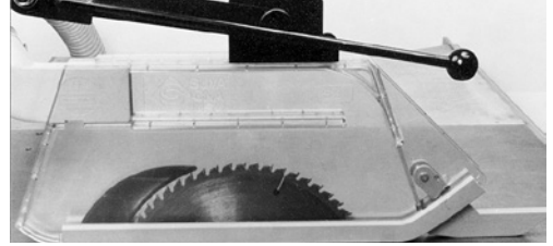
1 Parallel geführte Schutzhaube mit Vorritzblatt-Verdeckung.
