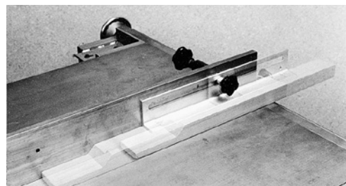
7 Verschiebbarer Anschlag
