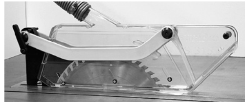
3 Am Spaltkeil montierte Schutzhaube.
