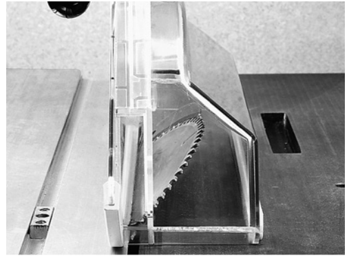
2 Auswechselbare, breite Schutzhaube.
