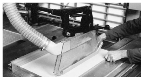
9 Absaugstutzen an der Schutzhaube
