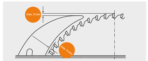
4 Korrekt eingestellter Spaltkeil.
