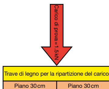
Figura 4 Esempio di prova per un ponteggio CC3 con carico utile 2,0 kN/m 2 e 2 piani larghi 30 cm.
