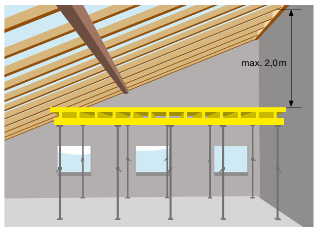
12 Fanggerüst unter einer Tragkonstruktion
