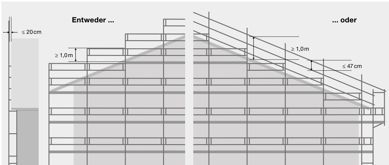
7 Fehlt an der Giebelseite der Spenglergang, darf der Abstand vom Seitenschutz zum Dachrand max. 20 cm betragen – die vertikale Höhe des Seitenschutzes beträgt dann mindestens 1,0 m.
