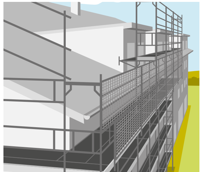
6 Das Fassadengerüst überragt den Dachrand der Gaube um mindestens 80 cm.
