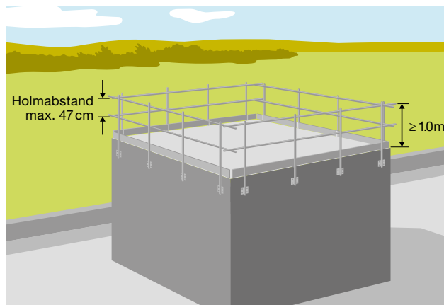
18 Permanenter Seitenschutz am Gebäude verankert
