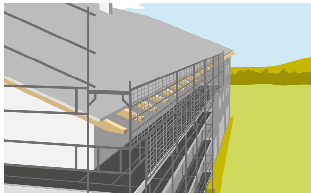
14 Lösung mit Innenkonsole am Gerüst. Sie verhindert, dass Personen zwischen Gerüst und Mauerwerk abstürzen.
