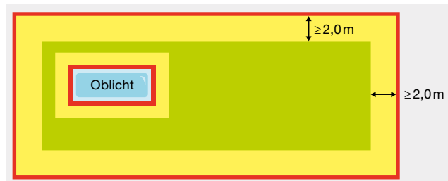
24 Gefahrenbereiche auf einem Flachdach
