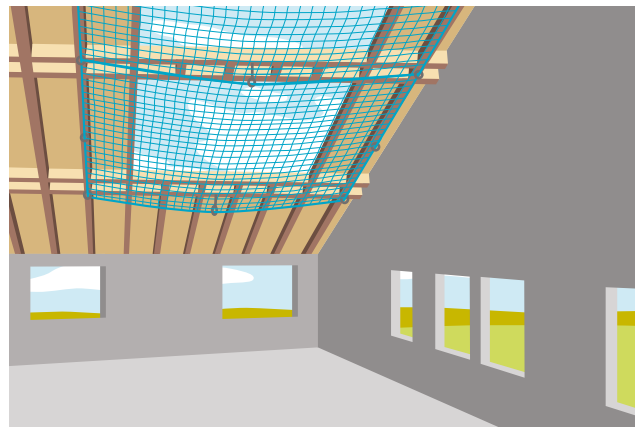
10 Auffangnetz bei der Öffnung fürs Dachfenster
