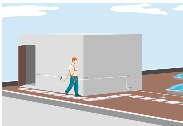
25 Sicherer Zugang auf ein Flachdach für Arbeiten von kurzer Dauer
