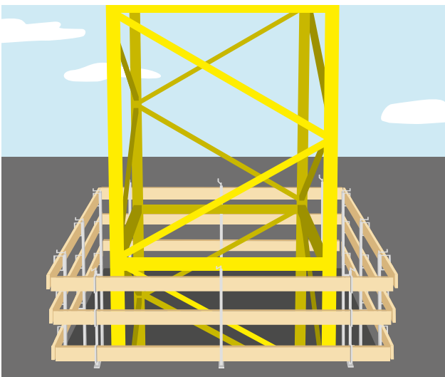
22 Dreiteiliger Seitenschutz um die Deckenöffnung herum
