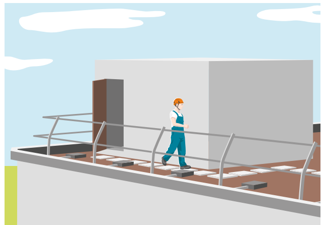
2 Kollektivschutz in der Nutzungsphase
