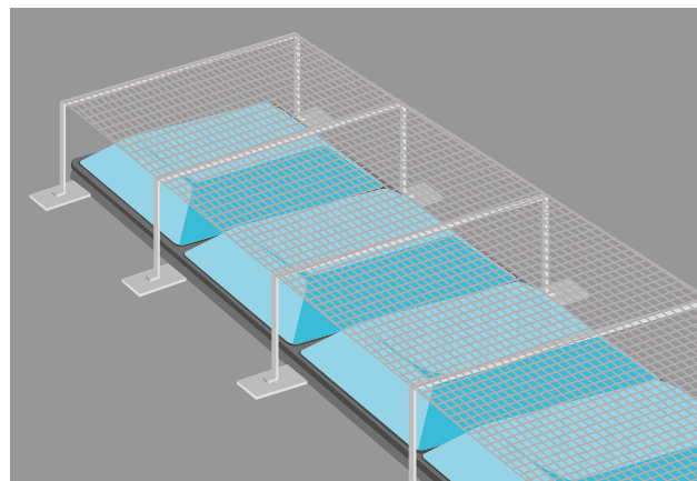
23 Kunststoffoblicht, mit Kollektivschutz (Gitterabdeckung) gesichert
