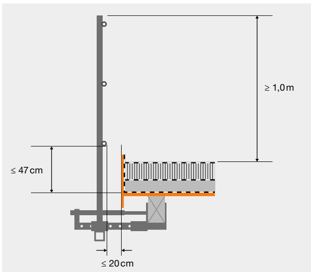
8 Giebelseitiger Seitenschutz (Querschnitt) mit zusätzlichem Rohr bei grossen Dämmungsstärken.
