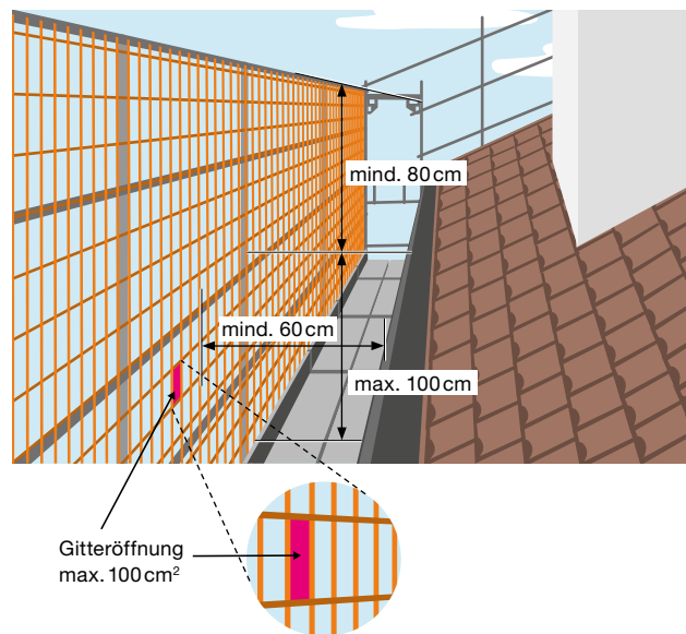
3 Spenglergang mit Dachdeckerschutzwand, Variante mit Gitter über die gesamte Höhe
