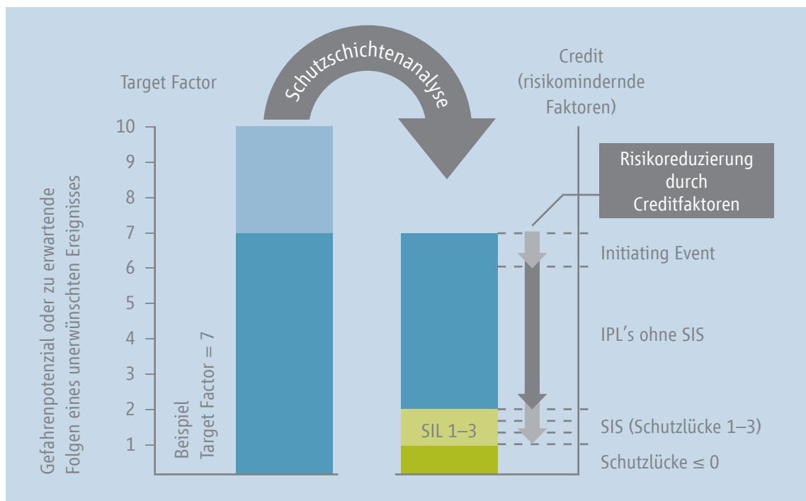
Abbildung 48: LOPA – Grundprinzip
