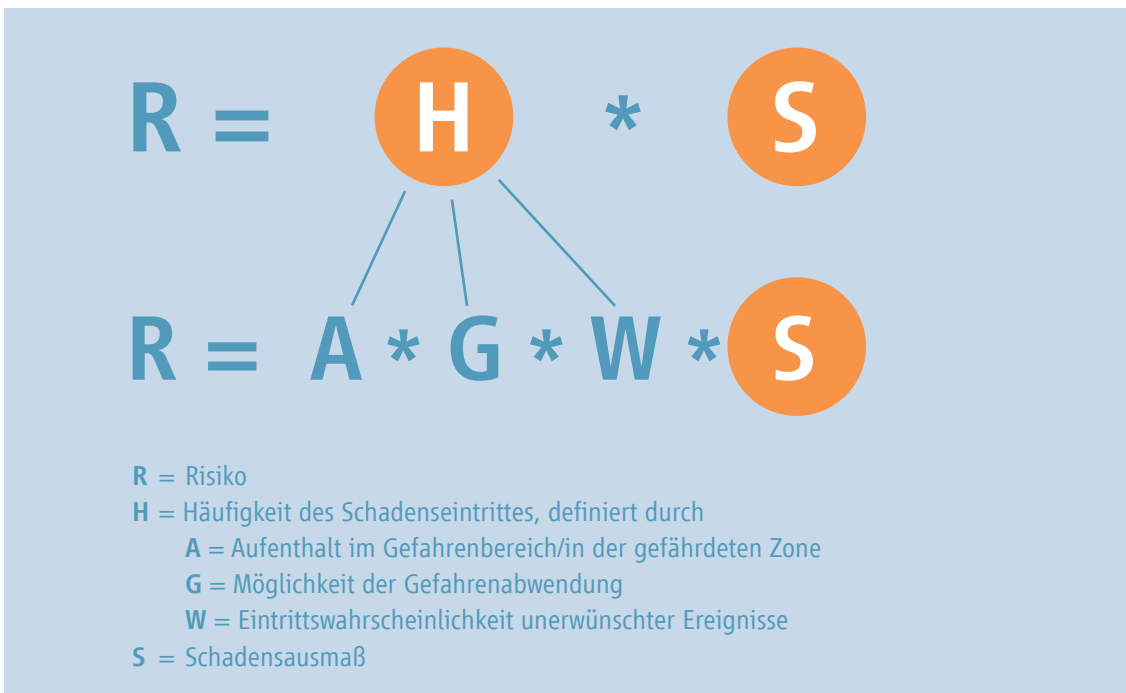
Abbildung 37: Risikodefinition gemäß Risikograph
