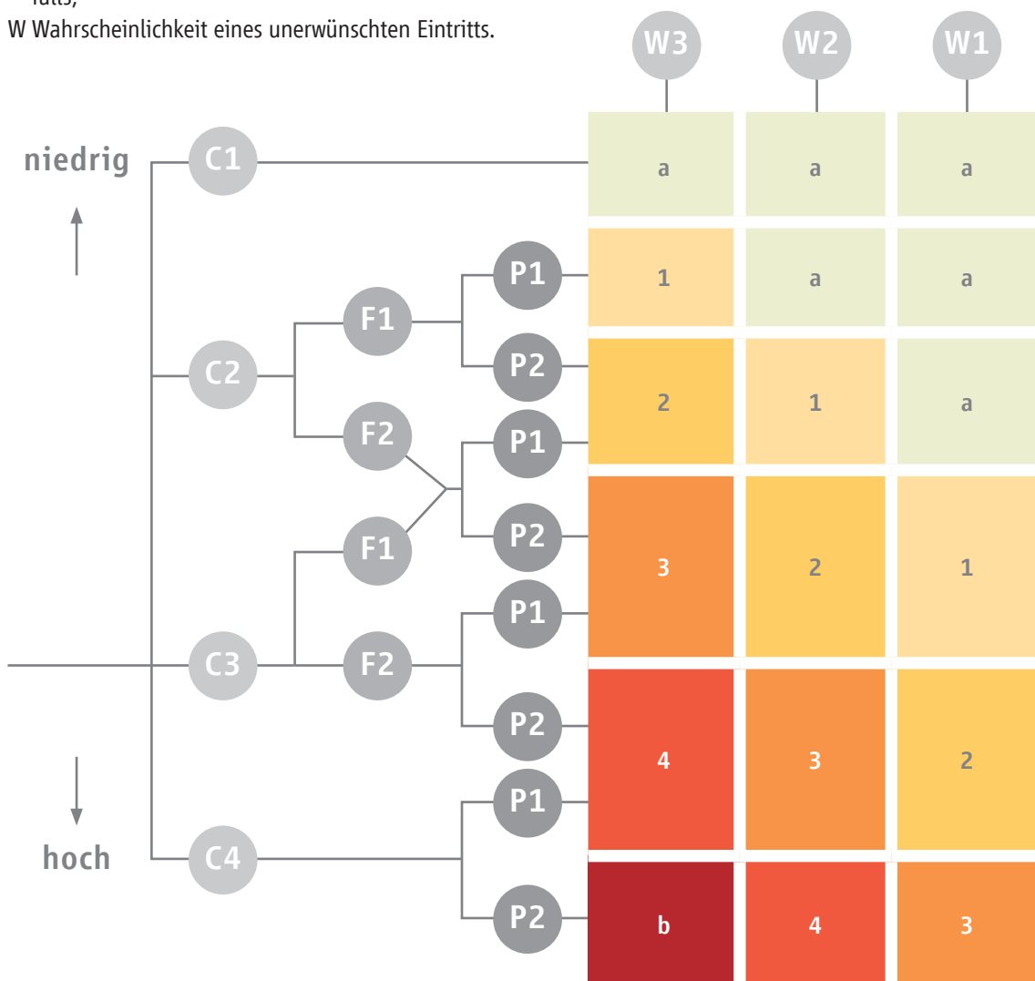
Abbildung 41: Risikograph gemäß DIN EN 50156-1 (Stand März 2016)
