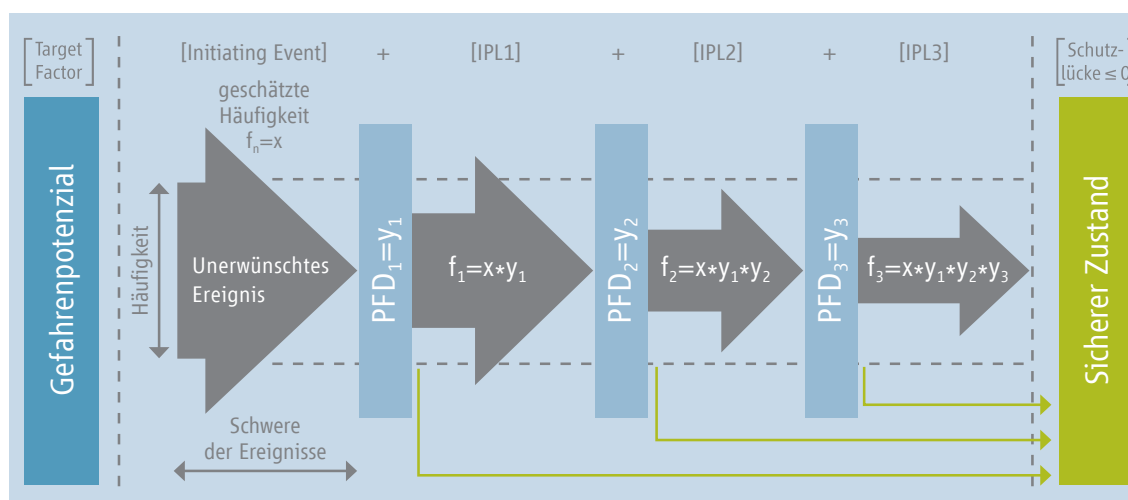
Abbildung 49: Konzept der LOPA unter Einbeziehung der Verfügbarkeit der einzelnen Schutzschichten
