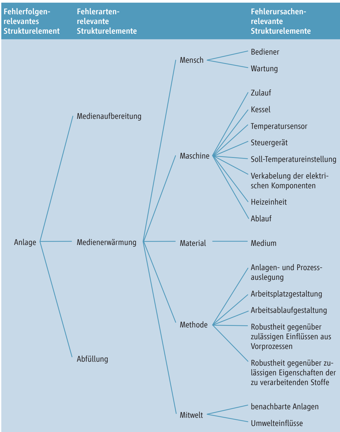
Abbildung 44: Strukturanalyse der FMEA bezogen auf eine einfache verfahrenstechnische Anlage
