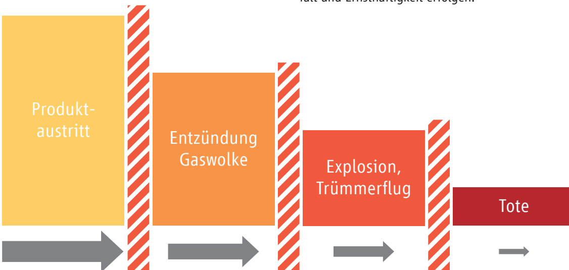
Abbildung 32: Visualisierung der Häufigkeit von Schadensszenarien am Beispiel des ungewollten Austritts eines brennbaren Mediums. Die Stärke des Pfeils symbolisiert die Wahrscheinlichkeit, die Barrieren die „conditional modifiers“
