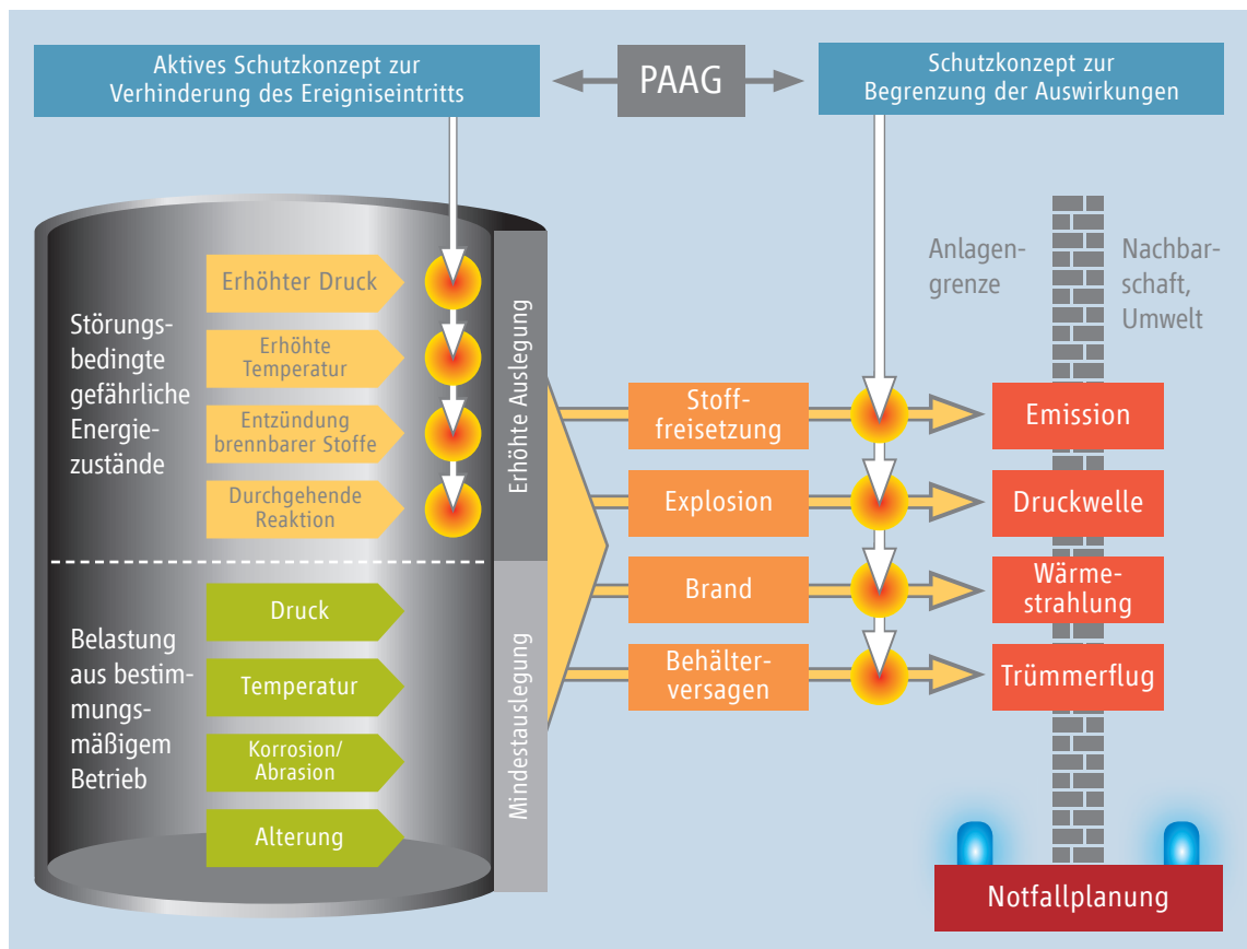
Abbildung 12: Typische Fragestellungen aus der Anwendung des PAAG/HAZOP-Verfahrens
