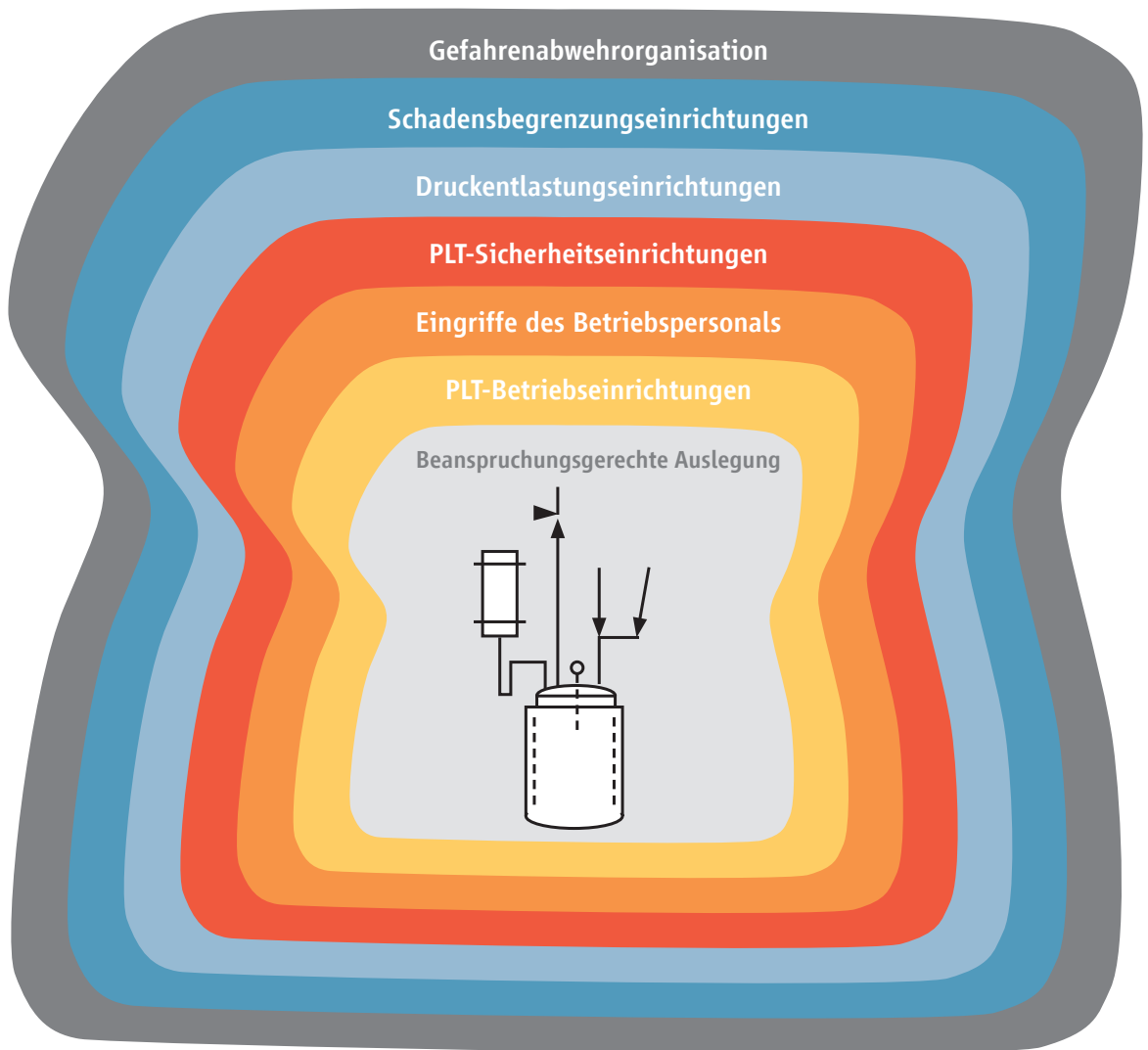
Abbildung 45: Modell der unabhängigen Schutzschichten
