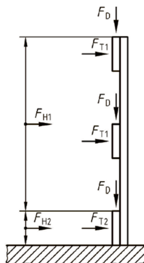
3 Forze esercitate sugli elementi della protezione laterale di classe A in base alla norma SN EN13374
