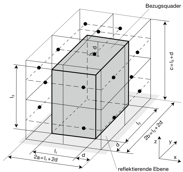
Bild 12 Beispiel einer Messfläche und der Mikrofonpositionen für eine mittelgrosse Maschine.
