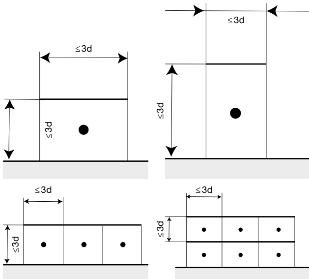
Bild 8 Festlegung der Mikrofonpositionen. d = Messabstand zum Bezugsquader.
