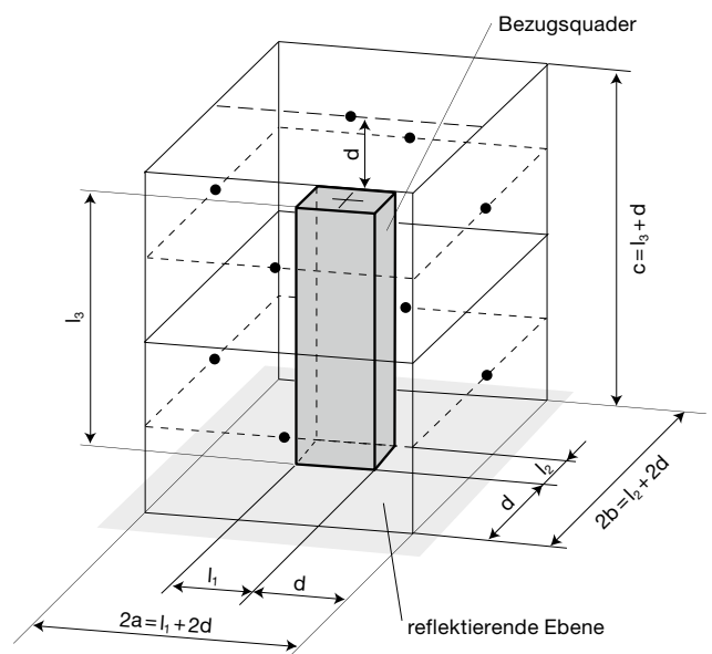
Bild 10 Beispiel einer Messfläche und der Mikrofonpositionen für eine hohe Maschine mit kleiner Grundfläche.
