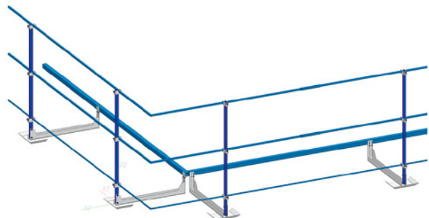
6 Garde-corps sans fixation à la toiture; stabilisé sur la structure de l'installation photovoltaïque
