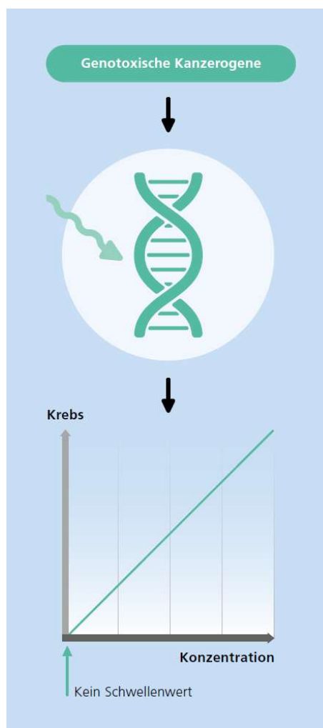
Fig. 2: substances cancérogènes sans seuil d'effet
