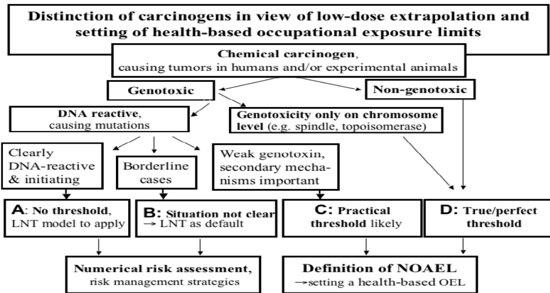
Fig. 5: évaluation des cancérrogènes selon le SCOEL [8]
