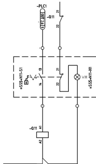
Bild 2: Revisionschalter, indirekt wirkend mit Meldeleuchte
