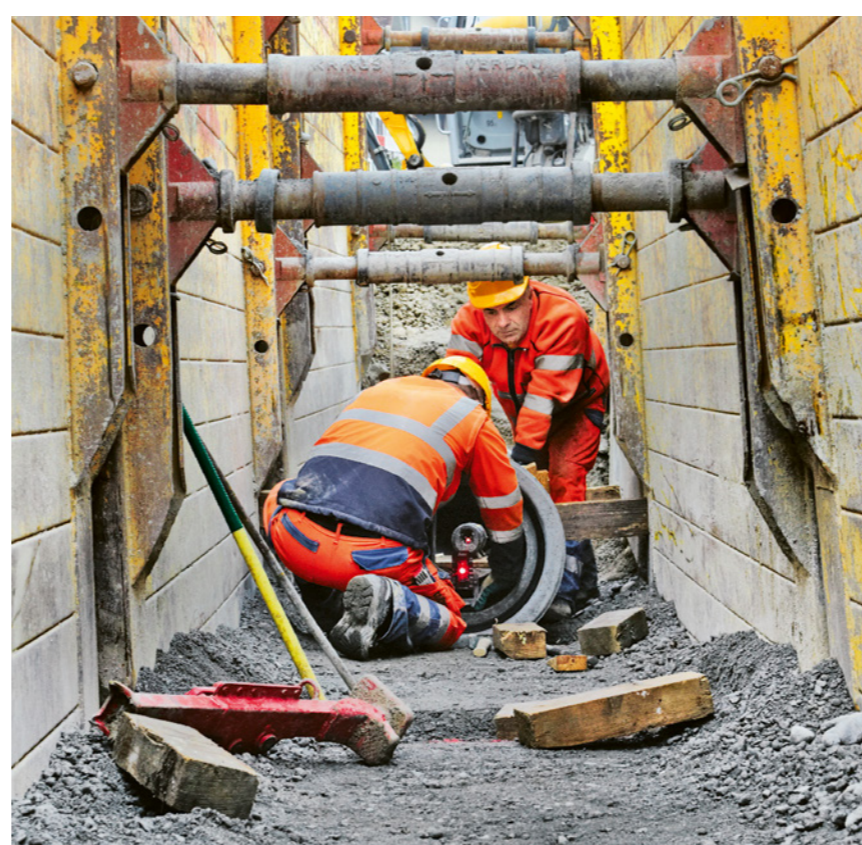
Regola 8: mettiamo in sicurezza gli scavi a partire da una profondità di 1,5m.
